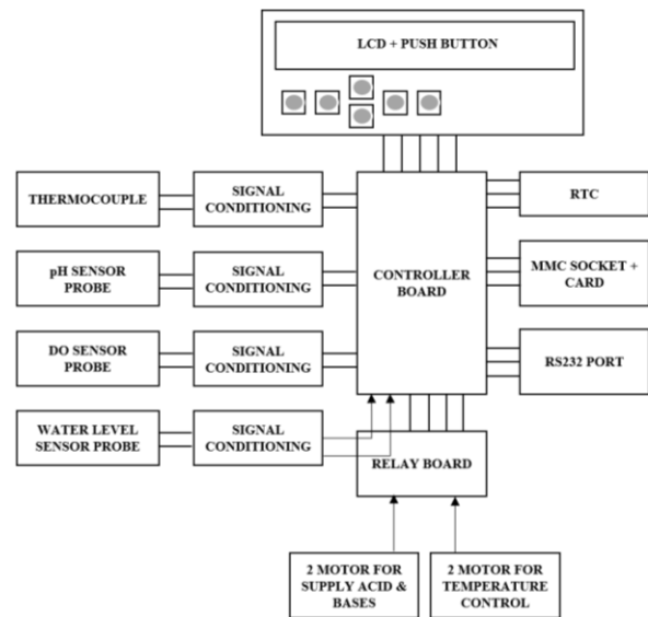
Gambar 1. Desain pengendalian kualitas air pada tambak ikan.
